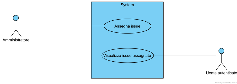
Figura 4: Use Case3 - Requisito funzionale 3.1.4 - Assegna issue e Requisito funzionale 3.1.7 - Visualizza issue assegnate
