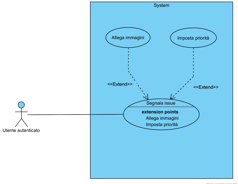
Figura 3: Use Case2 - Requisito funzionale 3.1.3 - Segnala issue
